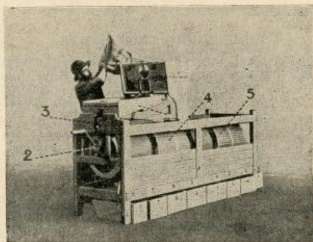
Сл. 36. Тријер „Маро“. 1. Покретно сито-тресалица. 2. Ручица за окретање са точићем. 3. Полука за тресалицу. 4. Сито за овас и јечам. 5. Сито за пшеницу и раж. 4. и 5. овална сита.
