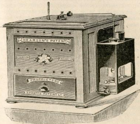
Сл 13. Машина за вештачко извођење. У употреби на живинарнику „Анђелка“ г. Р. Петровића, трг.
