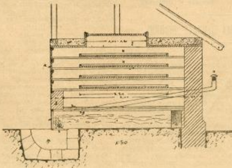
Слика 4. Уздужни пресјек кроз собицу преудешене босанске пушнице.
