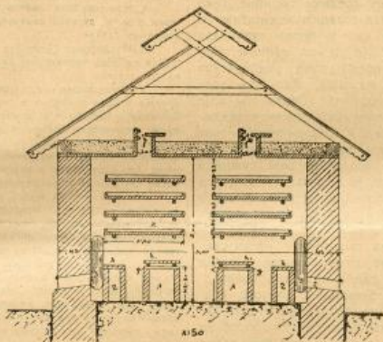
Слика 3. Попријечни пресјек преудешене босанске пушнице.
