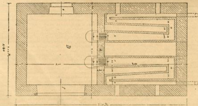
Слика 2. Темељни нацрт преуђене босанске пушнице.
