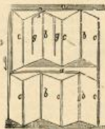
Сл. 6. Наводњавање попречним вадама са више одељења.
