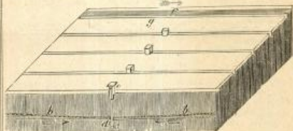
Сл. 9. Петерсов начин у хоризонталном пресеку.
