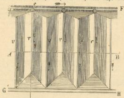
Сл. 3. Наводњавање уздужним вадама, основа водоравни вресекс.
