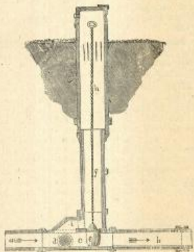
Сл. 8. Петерсов начин у вертикалном пресеку.
